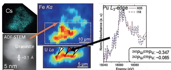
TEMとXRFマップが示すウラン酸化ナノ粒子とプルトニウムの局在。
