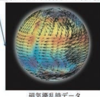
磁気擾乱時データ
