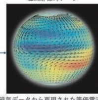
磁気データから再現された等価電流図
